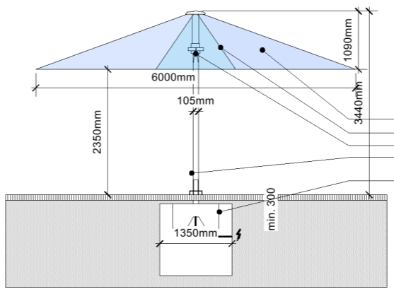
2 Parasol - Open Section Scale: 1:50
