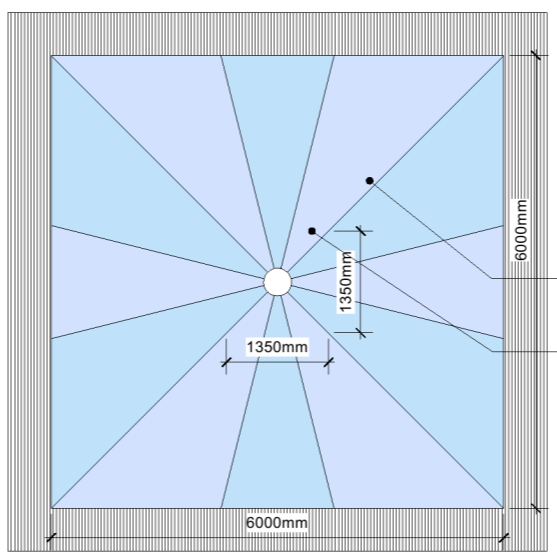
4 Parasol - Plan Scale: 1:50
